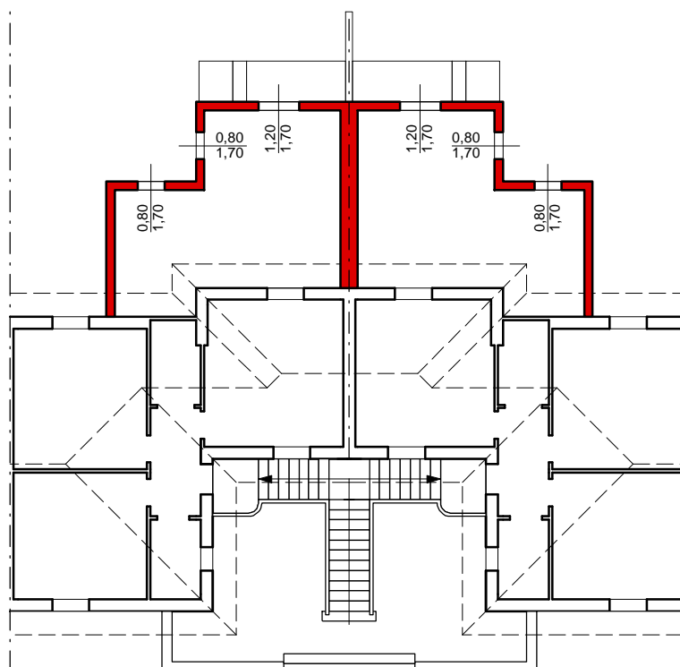
piano primo
